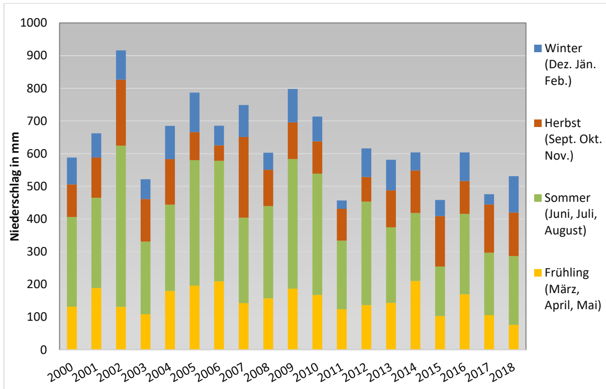
Abbildung 5: Niederschlagsmenge nach Jahreszeiten 2000-2018 - Messstation Kraftwerk Ottenstein
