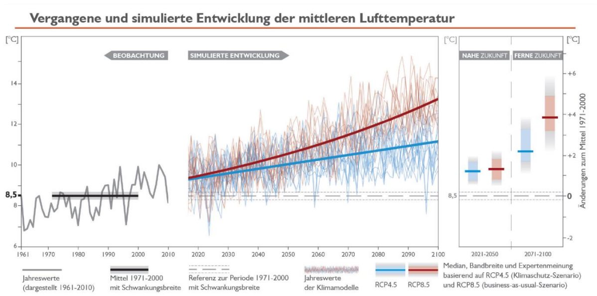
Abbildung 9: Entwicklung der mittleren Lufttemperatur in NÖ (ÖKS15)
