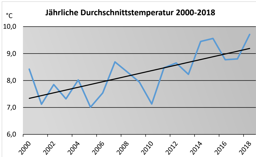
Abbildung 2: Jährliche Durchschnittstemperatur 2000-2018 - Messstation Kraftwerk Ottenstein
