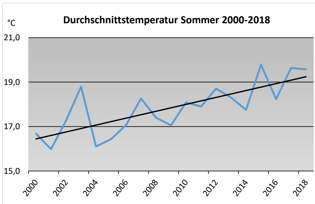
Abbildung 3: Durchschnittstemperatur im Sommer 2000-2018 - Messstation Kraftwerk Ottenstein
