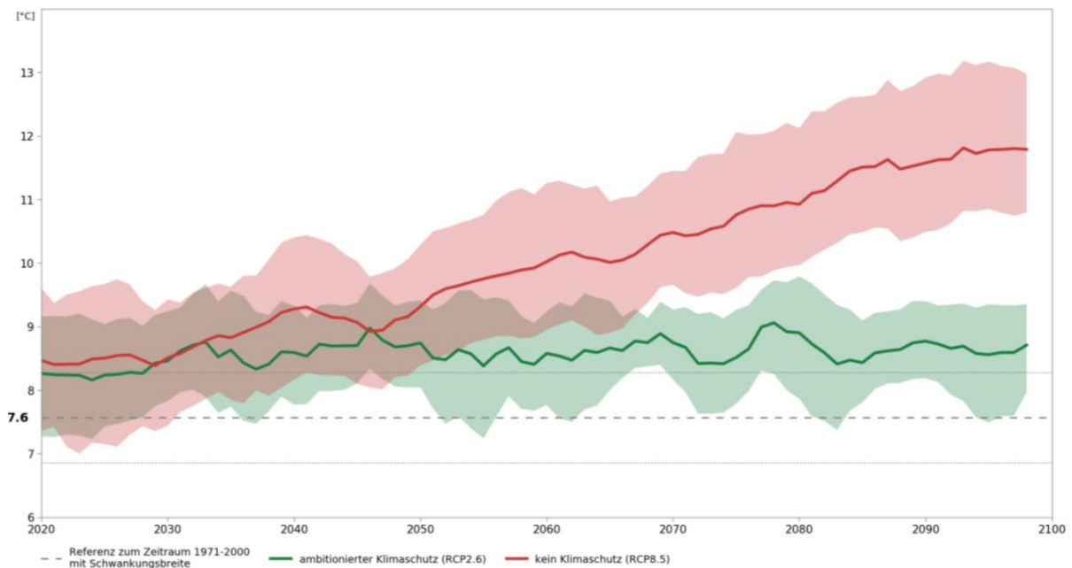
Abbildung 10: Zukünftige Entwicklung der mittleren Jahrestemperatur in der Region Kampseen (ZAMG, 2019)
