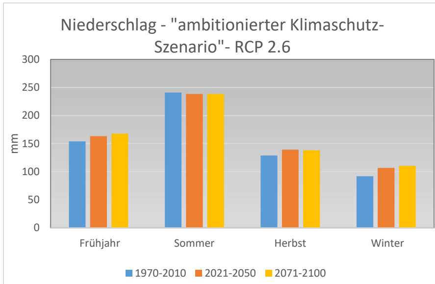
Abbildung 16: Entwicklung des Niederschlags – „ambitionierter Klimaschutz-Szenario“ – Region Kampseen (ZAMG, 2019)
