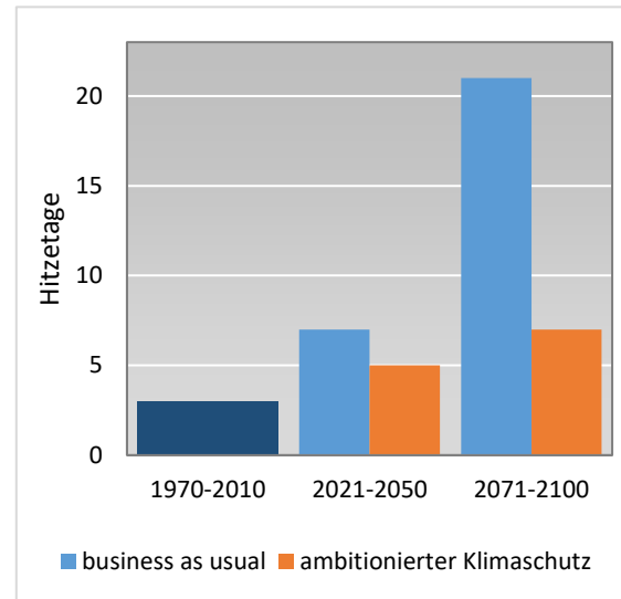
Abbildung 12: Entwicklung der Hitzetage in der Region Kampseen (ZAMG, 2019)
