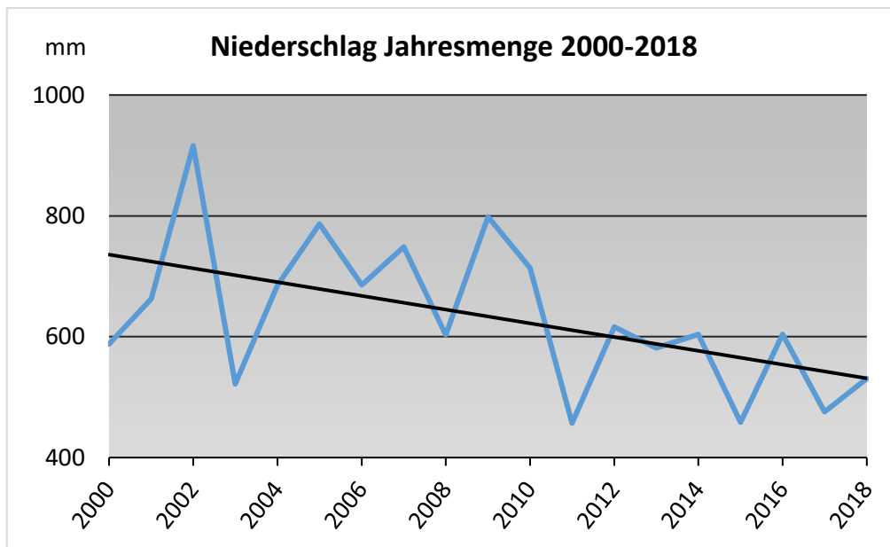
Abbildung 4: Niederschlag Jahresmenge 2000-2018 - Messstation Kraftwerk Ottenstein
