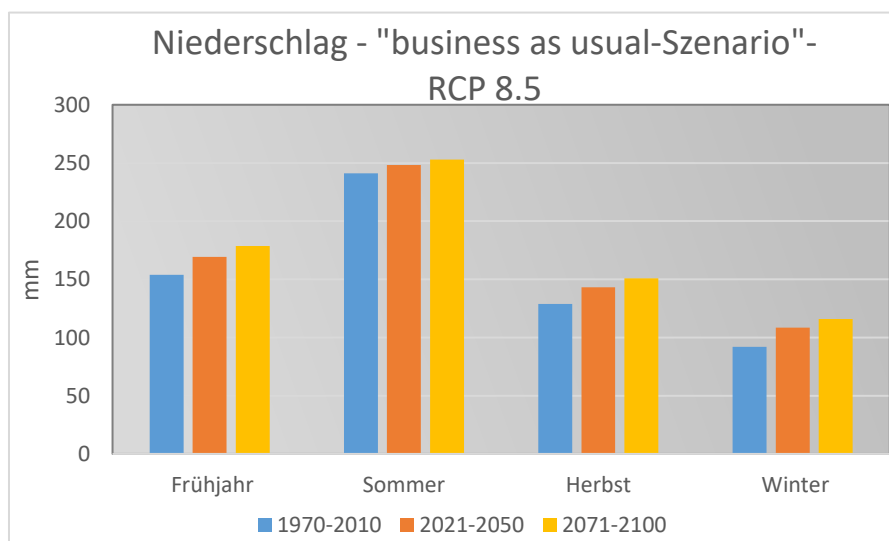
Abbildung 15: Entwicklung des Niederschlags – „business as usual-Szenario“ – Region Kampseen (ZAMG, 2019)
